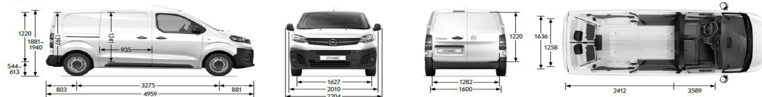
Vivaro Cargo M Alle Maße in mm
