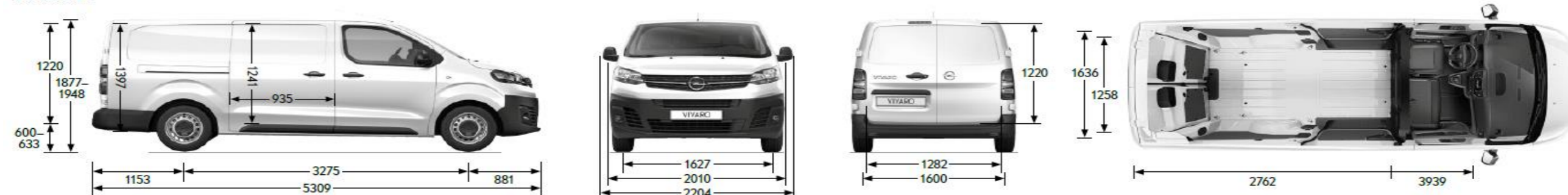
Vivaro Cargo L Alle Maße in mm
